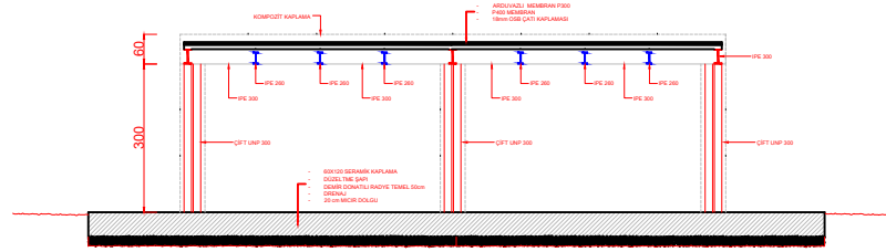
A -A KESİTİ
